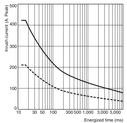
G3PB-535B-VD, G3PB-545B-VD
