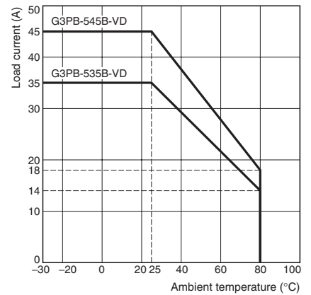
G3PB-535B-VD, G3PB-545B-VD
