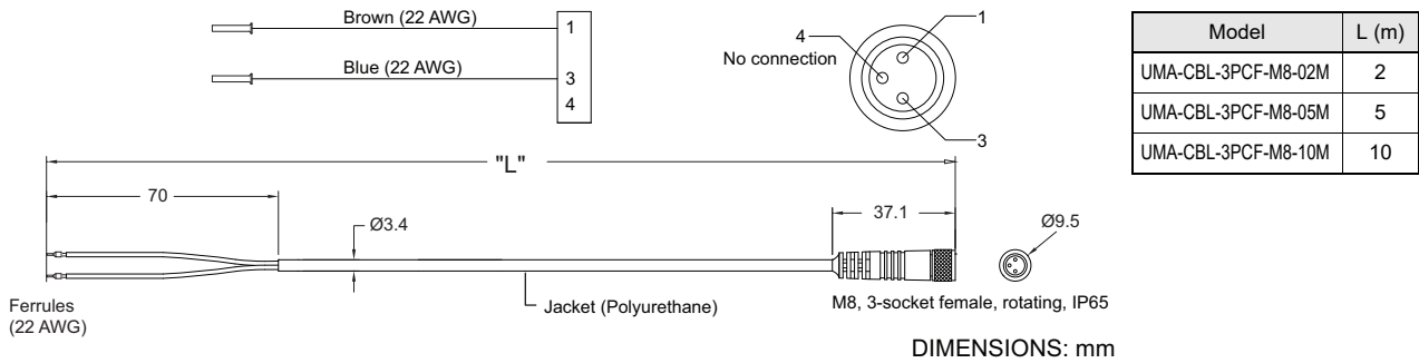
Fig. 6-3 UMA-CBL-3PCF-M8-□M
