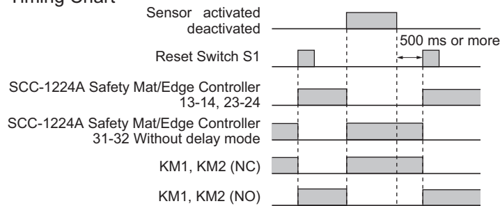
Fig. 3-13 UMA with SCC-1224A (Manual Reset Mode)
