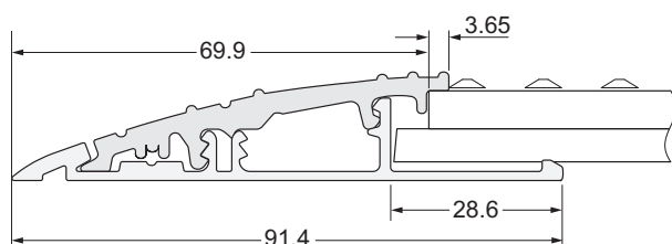
Fig. 4-1 UMRT□
