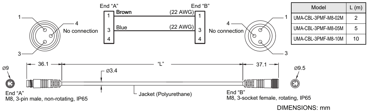
Fig. 6-4 UMA-CBL-3PMF-M8-□M
