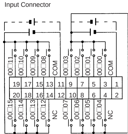
CPM2B-32EDR CPM2B-32EDT/32ED1T
