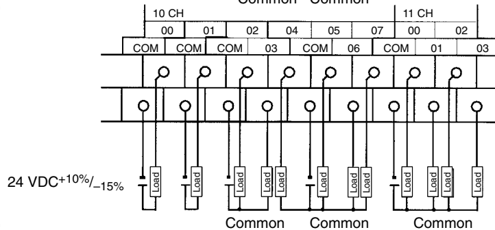
CPM1A-30CDT-□(-V1)
